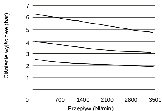
Charakterystyki regulacji
