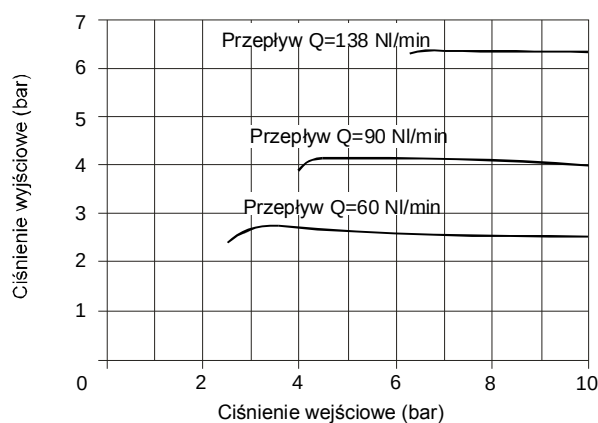
Charakterystyki regulacji
