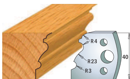
Para noży 690.103 Para ograniczników 691.103
