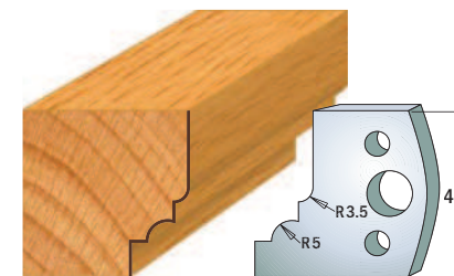
Para noży 690.020 Para ograniczników 691.020
