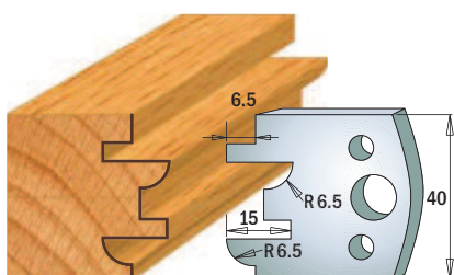
Para noży 690.096 Para ograniczników 691.096
