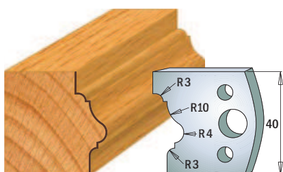
Para noży 690.102 Para ograniczników 691.102
