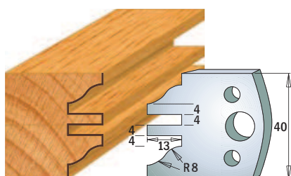
Para noży 690.097 Para ograniczników 691.097
