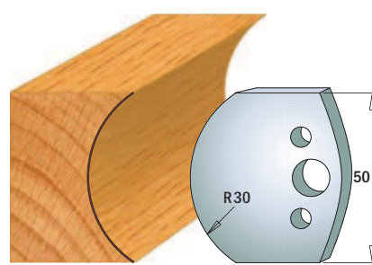
Para noży 690.544 Para ograniczników 691.544
