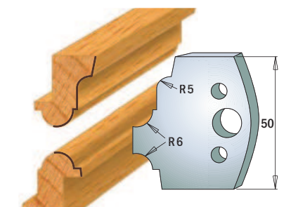
Para noży 690.542 Para ograniczników 691.542
