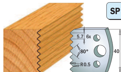
Para noży 690.077 Coppia di limitator/Par contracuchillas 691.077
