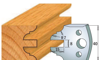
Para noży 690.099 Para ograniczników 691.099
