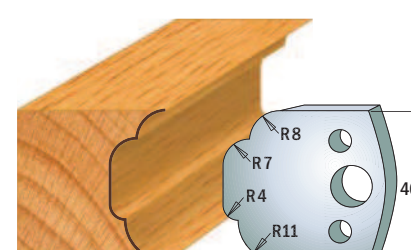
Para noży 690.023 Para ograniczników 691.023
