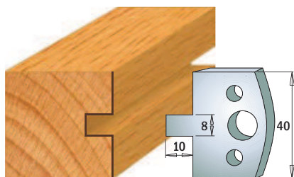
Para noży 690.094 Para ograniczników 691.094
