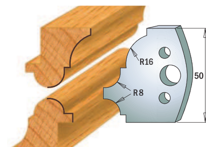
Para noży 690.541 Para ograniczników 691.541
