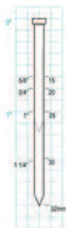
LNF - 32AC
