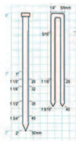
LU - 50FAC
