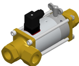
Handnotbetätigung manual override mechanische Option = 08 mechanical option = 08
